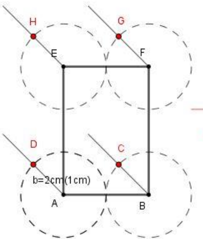
Bočné hrany Z každého vrcholu zostrojíte kružnicu s polomerom bočnej hrany skrátenej o polovicu skutočnej veľkosti.
